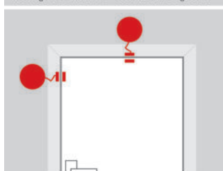
Montage neben der Tür – Reedkontakt abgesetzt
