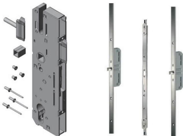
Stulp-Garnitur: RS 1300: mit Rundbolzen
